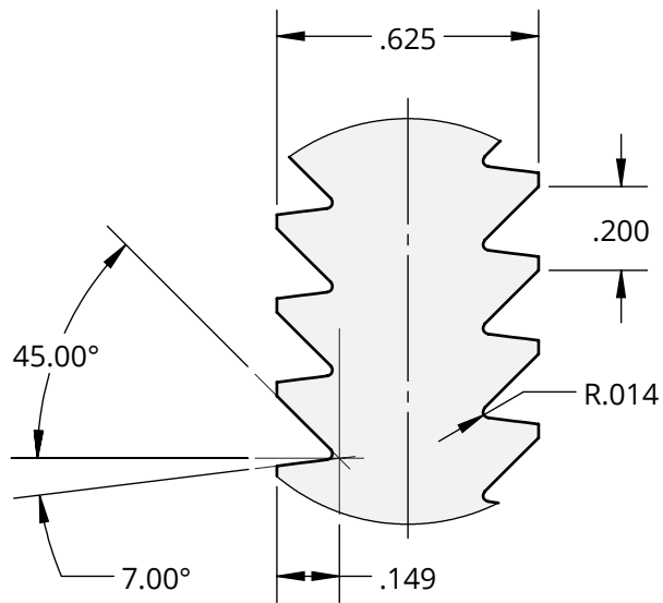
Bolt
