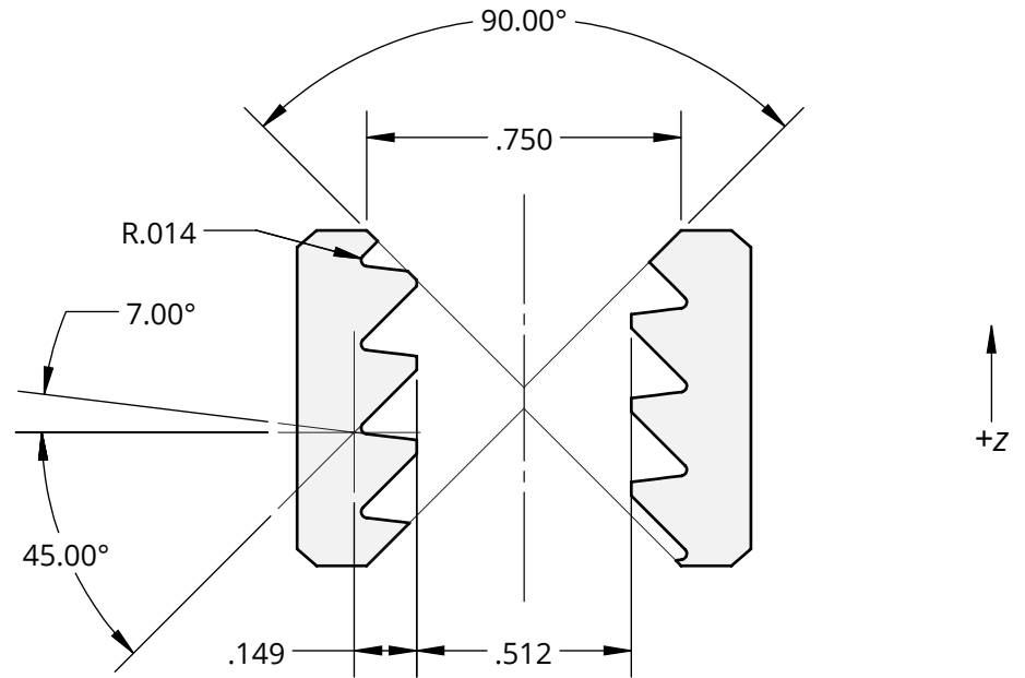
Nut
